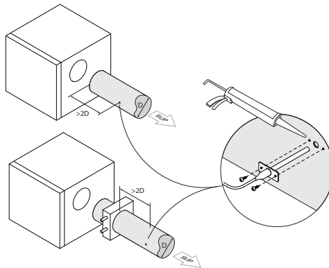
15b pav. Tiekiamo oro temperatūros jutiklio montavimas
