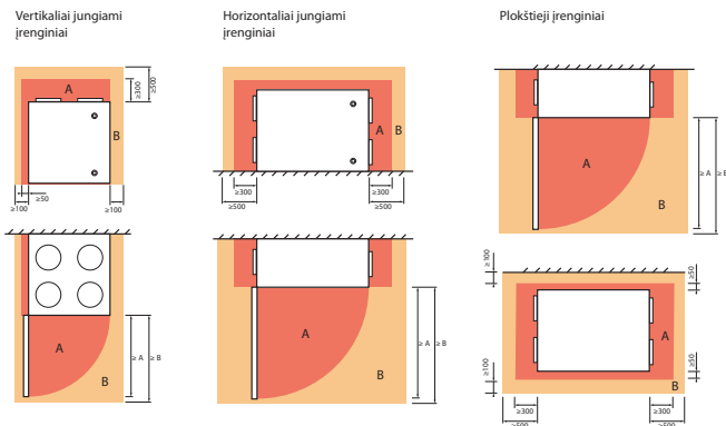
5 pav. Minimali erdvė įrenginio priežiūrai
