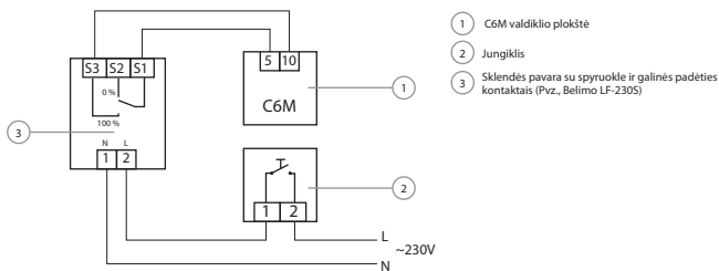
16 pav. „Pirmenybės“ vėdinimo režimo įjungimo pavyzdys, kai naudojamas papildomas oro ištraukimas su motorizuota sklendė (žr. 10 pav.)
