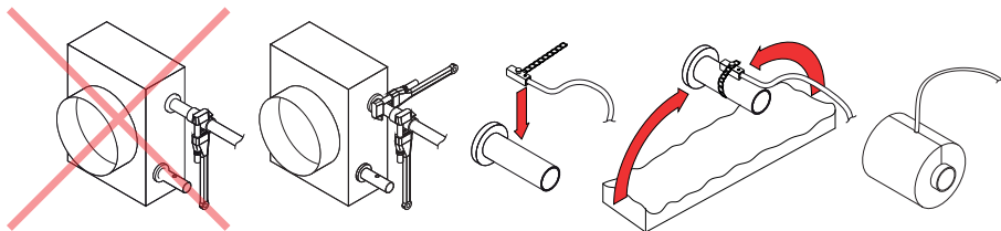
11 pav. Vandens šildytuvo/aušintuvo atvamzdžių prijungimas ir vandens temperatūros jutiklio montavimas
