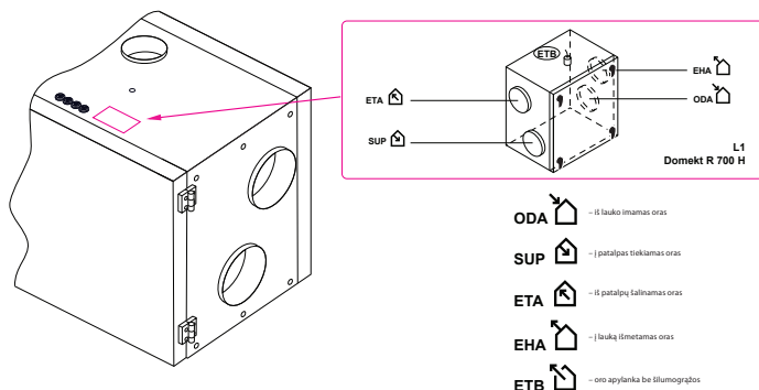
9 pav. Ortakių žymėjimas
