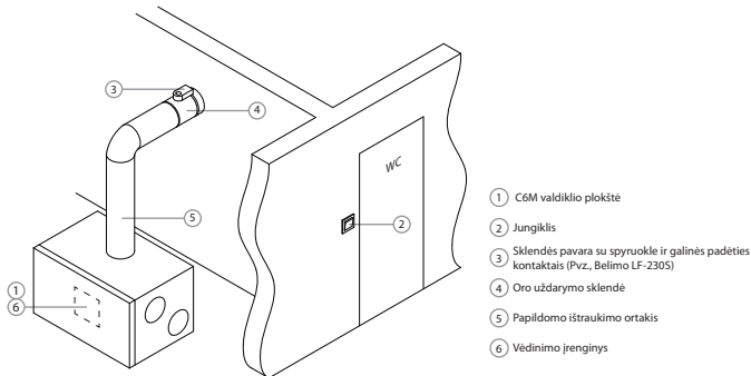
10 pav. Papildomo oro ištraukimo ortakio montavimo pavyzdys
