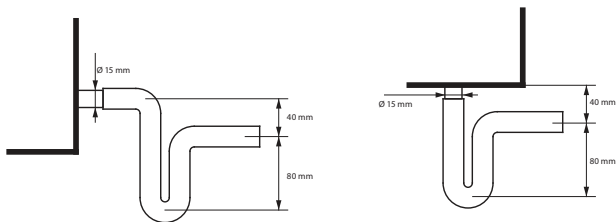
12a pav. Sifono be atbulinio vožtuvo montavimas
