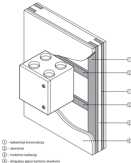
8 pav. Įrenginio tvirtinimas ant gipso kartono pertvaros
