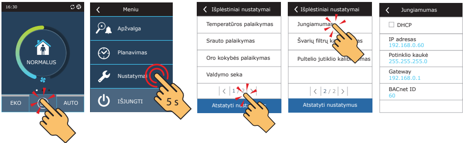
19 pav. Vėdinimo įrenginio IP adreso peržiūra ir keitimas pultelyje
