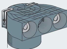
classic Luftdurchlass plus 90° classic outlet plus 90° NW 63 Art. Nr. 78363382
