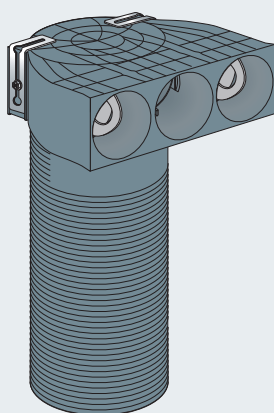
classic Luftdurchlass plus 90° classic outlet plus 90° NW 63 Art. Nr. 78363381
